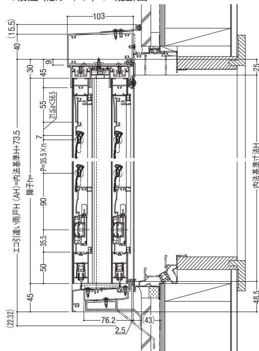
4枚建 (窓タイプ) / 縦断面
