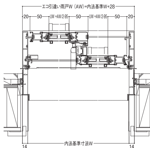
2枚建・4枚建共通 / 横断面
