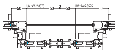
4枚建 / 横断面 (召合せ部)
