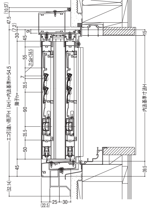
4枚建 (窓タイプ) / 縦断面
