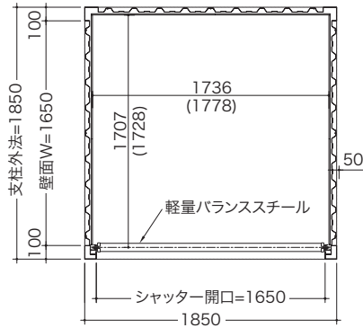
【平面図】1坪タイプ (内寸法はSB-10(内装レス)タイプを示す。)
