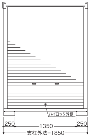
【正面図】1坪タイプ
