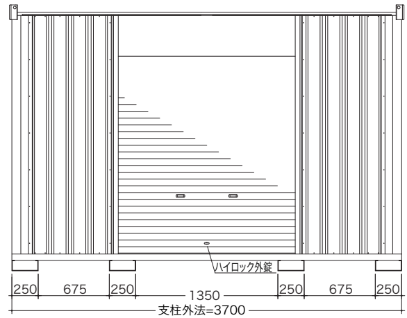
【正面図】2坪タイプ
