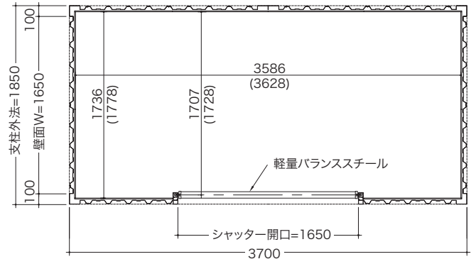
【平面図】2坪タイプ (内寸法はSB-20(内装レス)タイプを示す。)
