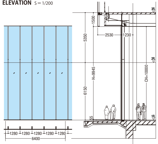
ELEVATION S=1/200
