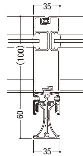
既存方立 (例)
