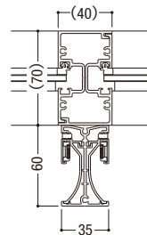
既存方立 (例)
