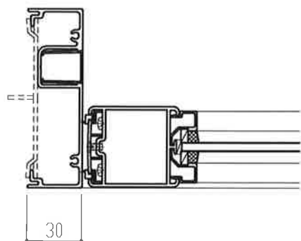
RC枠
