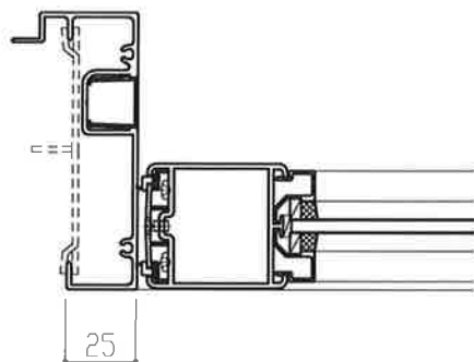
ALC枠
