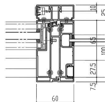
連窓方立パターン⑧
