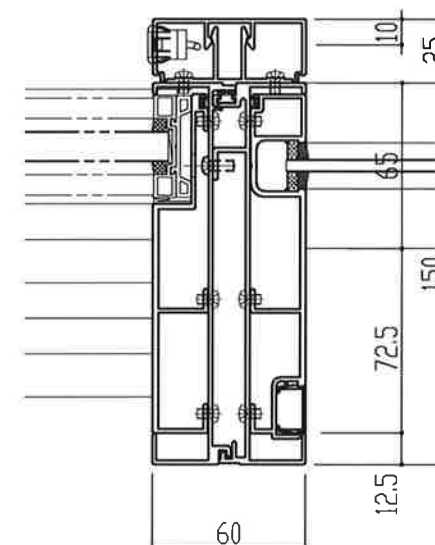
組方立パターン⑫
