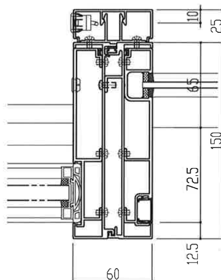
組方立パターン⑩
