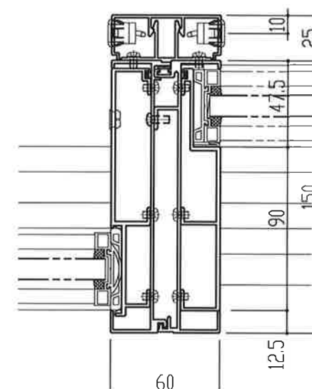
組方立パターン④
