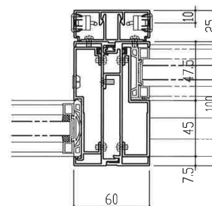
連窓方立パターン④
