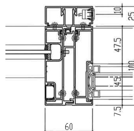
連窓方立パターン⑦
