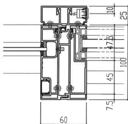
連窓方立パターン⑤
