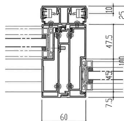
連窓方立パターン③
