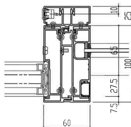
連窓方立パターン⑥
