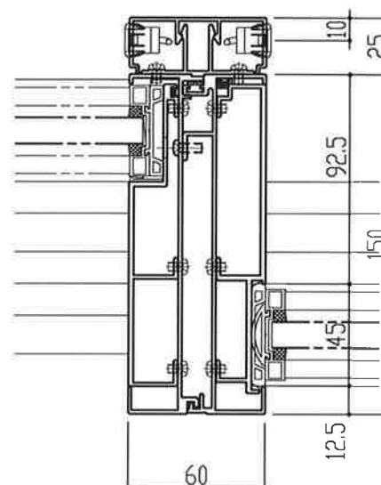
組方立パターン③
