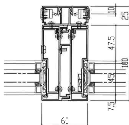
連窓方立パターン①
