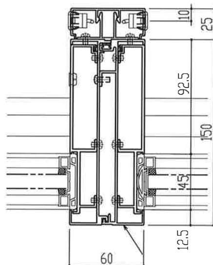
組方立パターン①
