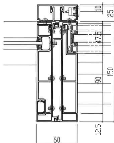
組方立パターン⑨
