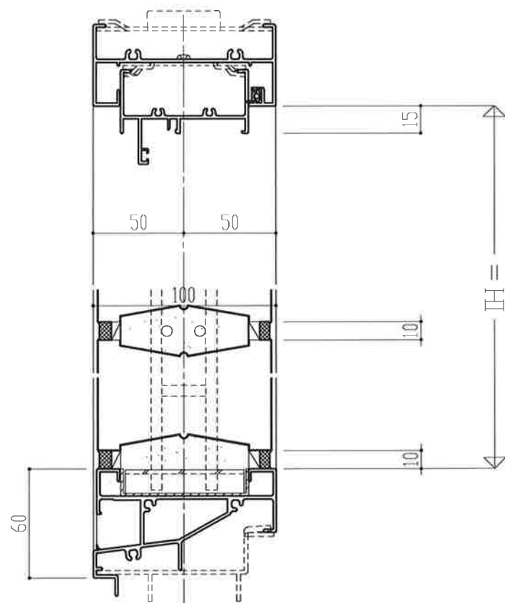
FIX窓 RC枠
