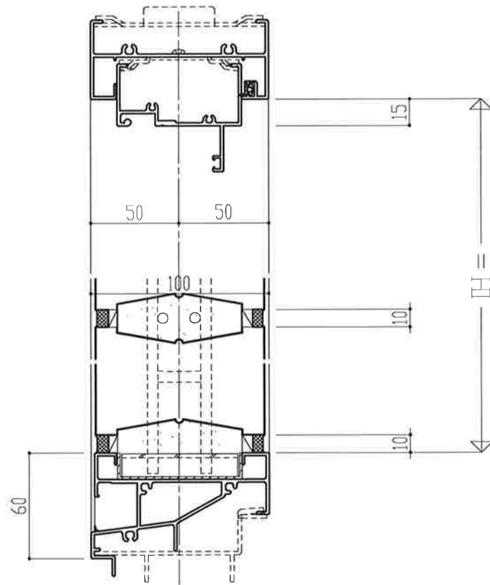
突出し排煙窓 RC枠
