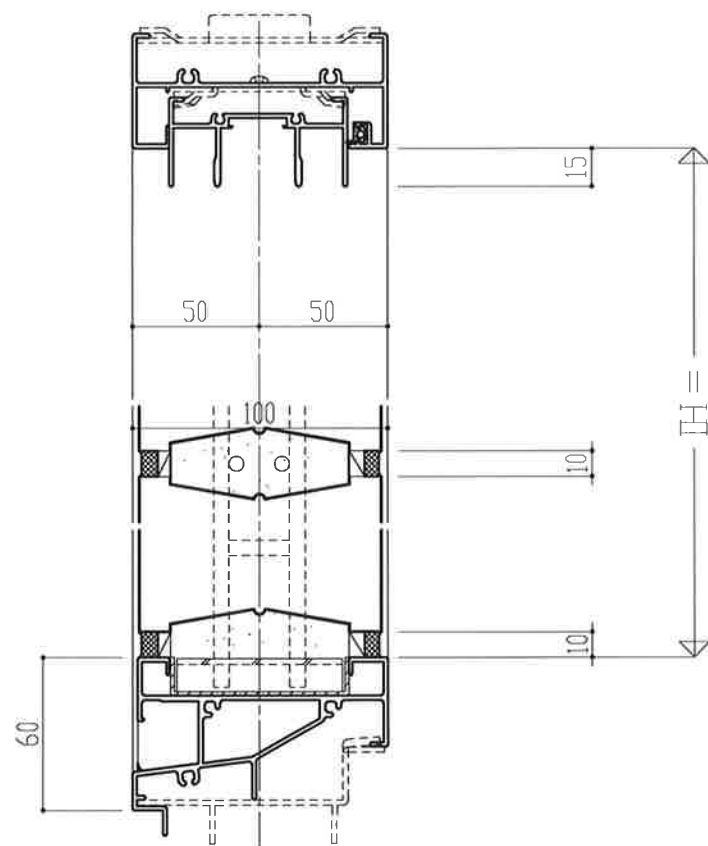
引違い窓 RC枠
