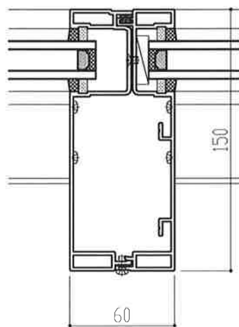
②150mm見込み方立
