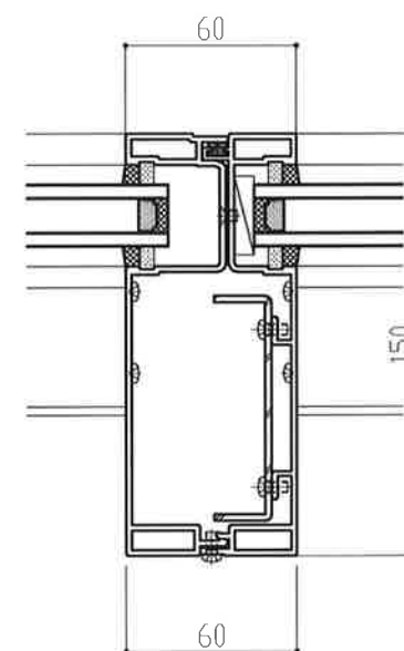
150mm方立
