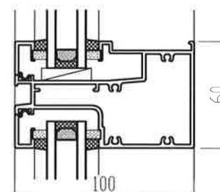
③100mm見込み無目
