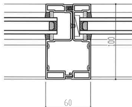
①100mm見込み方立
