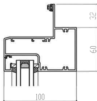
⑤100mm見込み無目
