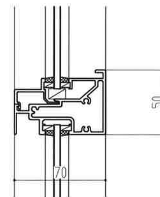
⑤70mm見込み無目
