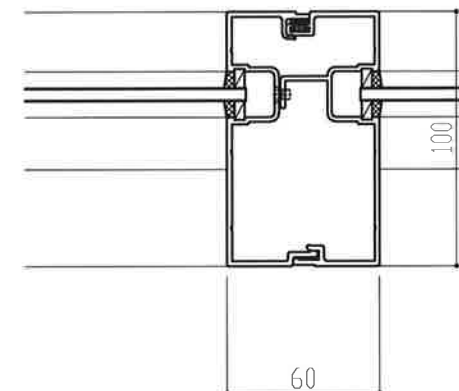
⑪100mm見込み方立
