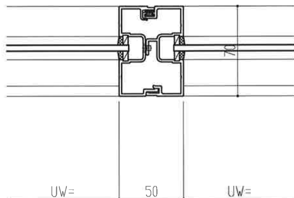
組合せ方立(70mm見込み)
