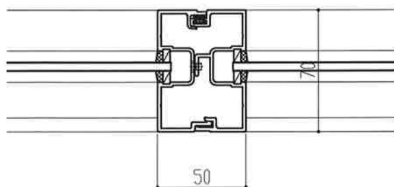
⑥70mm見込み方立
