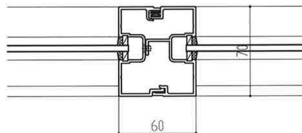
⑦70mm見込み方立
