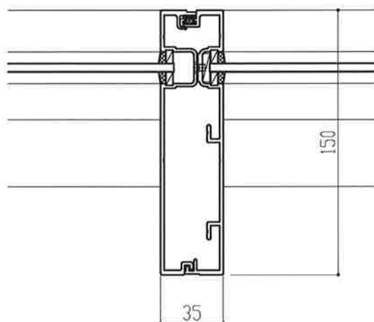
⑨150mm見込み方立
