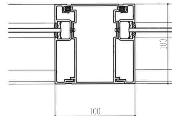
⑪100mm見込み方立
