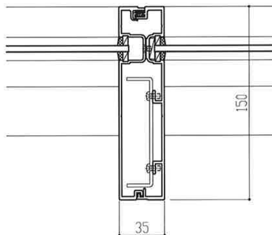
⑩150mm見込み方立
