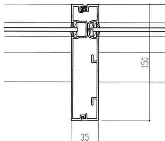
③150mm見込み方立
