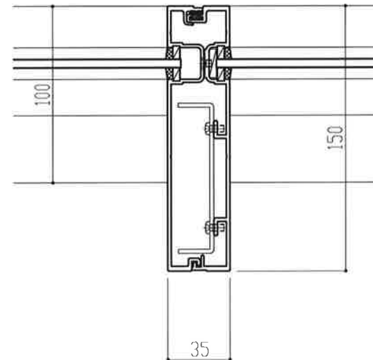
組合せ方立(回転取付タイプ) (150mm見込)
