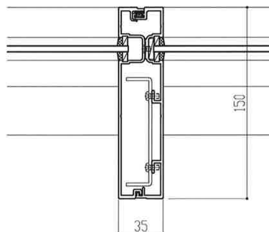
④150mm見込み方立
