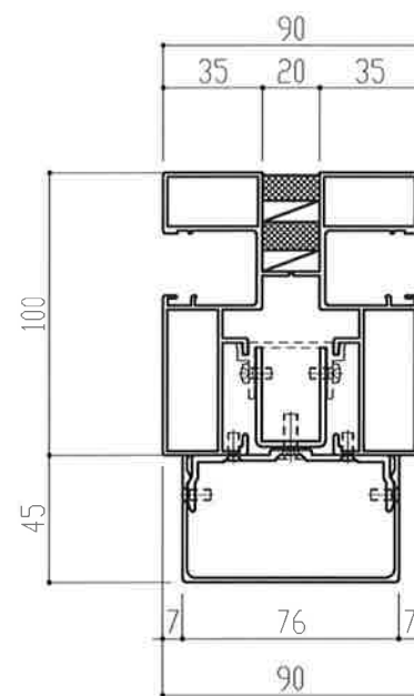
フロント連窓方立(非防火)
