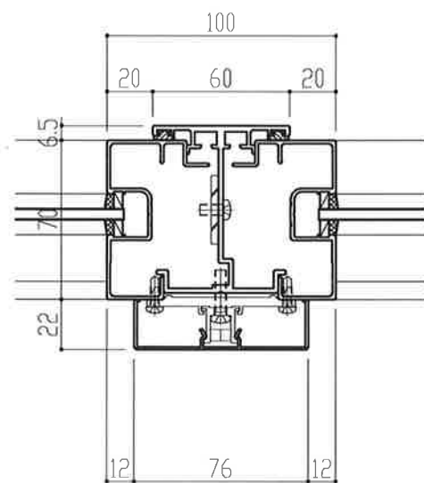
ALC方立
