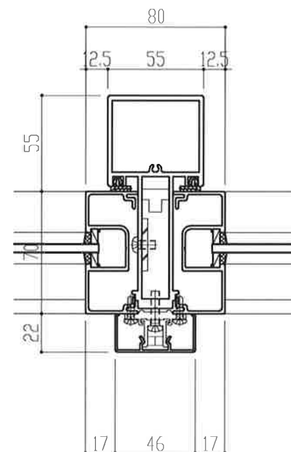
B方立
