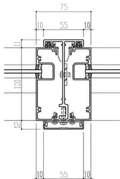
100mm枠
