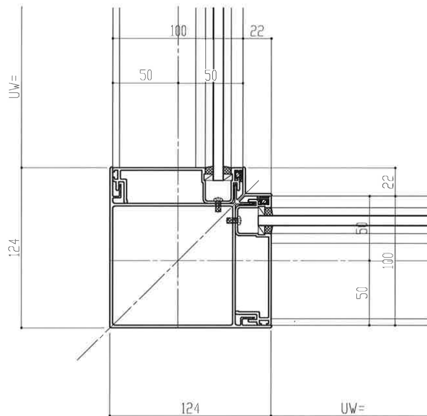
入隅
