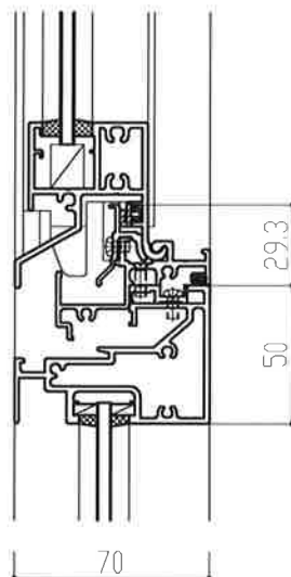
①70mm見込み FIX
