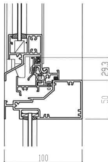
②100mm見込み FIX
