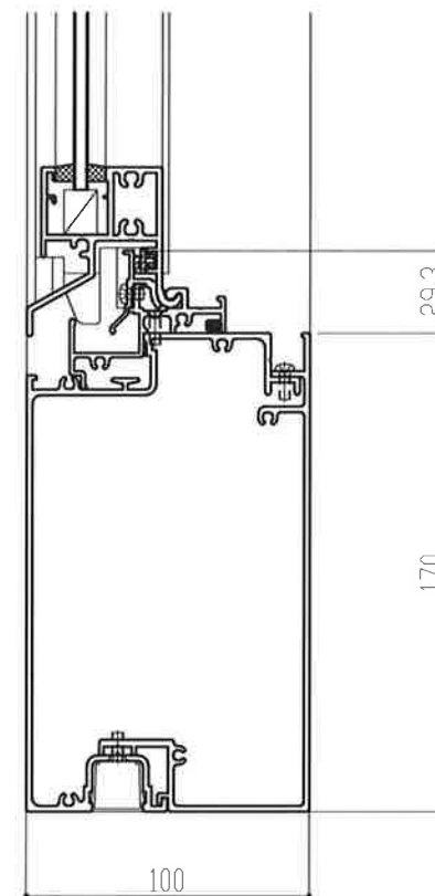
③100mm見込み FIX
