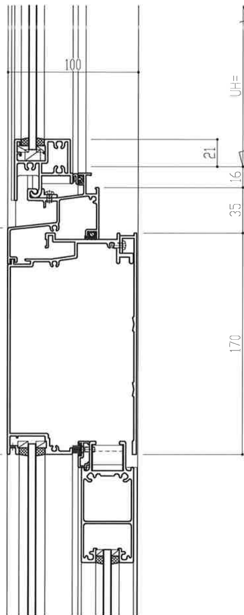
外倒し排煙窓/自動ドア
