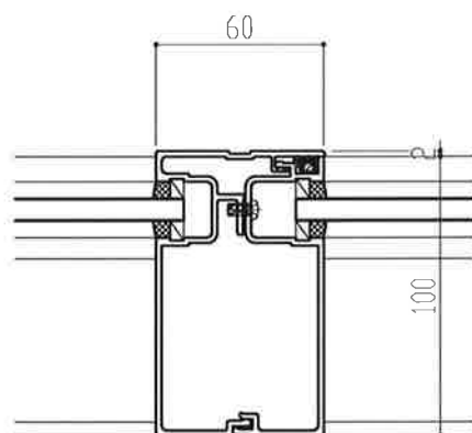
①80mm見付・水密方立
