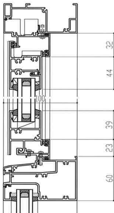
外倒し排煙窓-FIX
