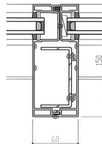
④150mm見込み方立 St補強付
