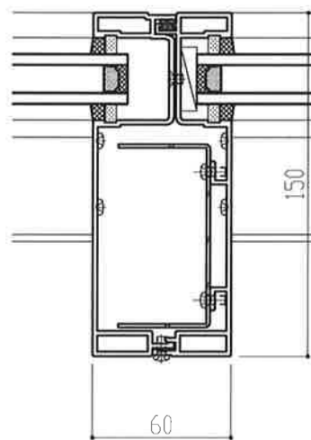
②150mm見込み方立 St補強付
