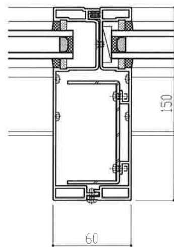
③150mm見込み方立 St補強付
