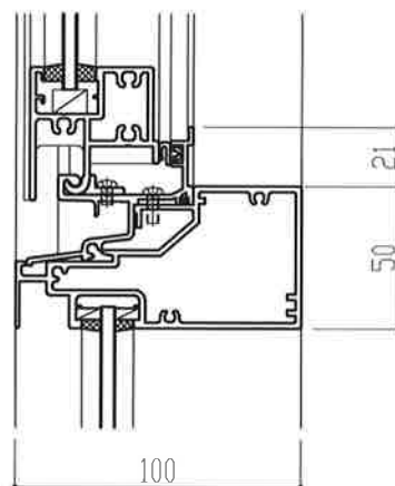
②100mm見込み FIX
