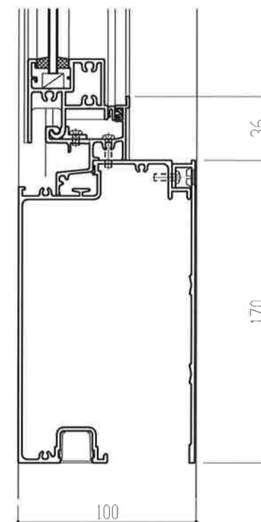
⑦100mm見込み 自動ドア
