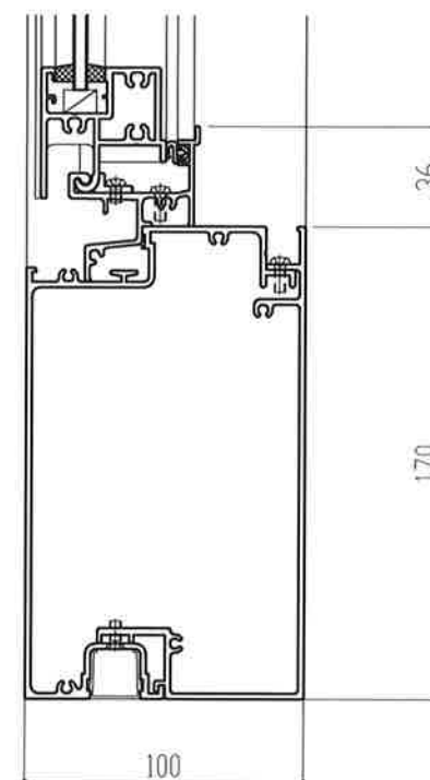
③100mm見込み FIX
