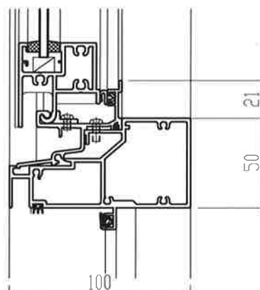
⑤100mm見込み 框ドア
