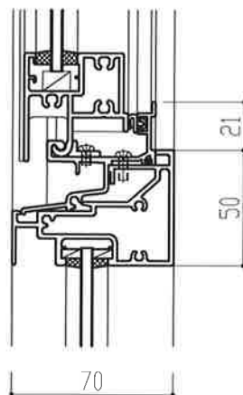
①70mm見込み FIX
