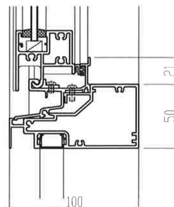
⑥100mm見込み フロアヒンジドア
