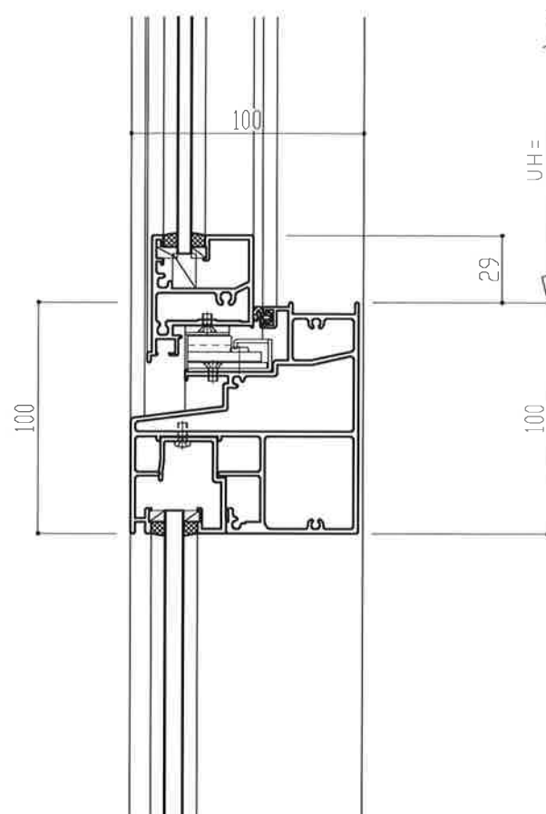
FIX無目 たてすべり出ノFIX
