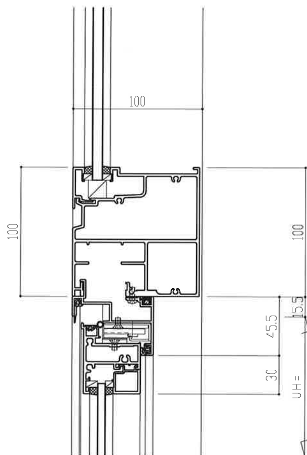
FIX無目 FIXノたてすべり出
