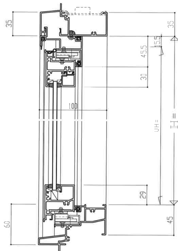
障子：Aタイプ
