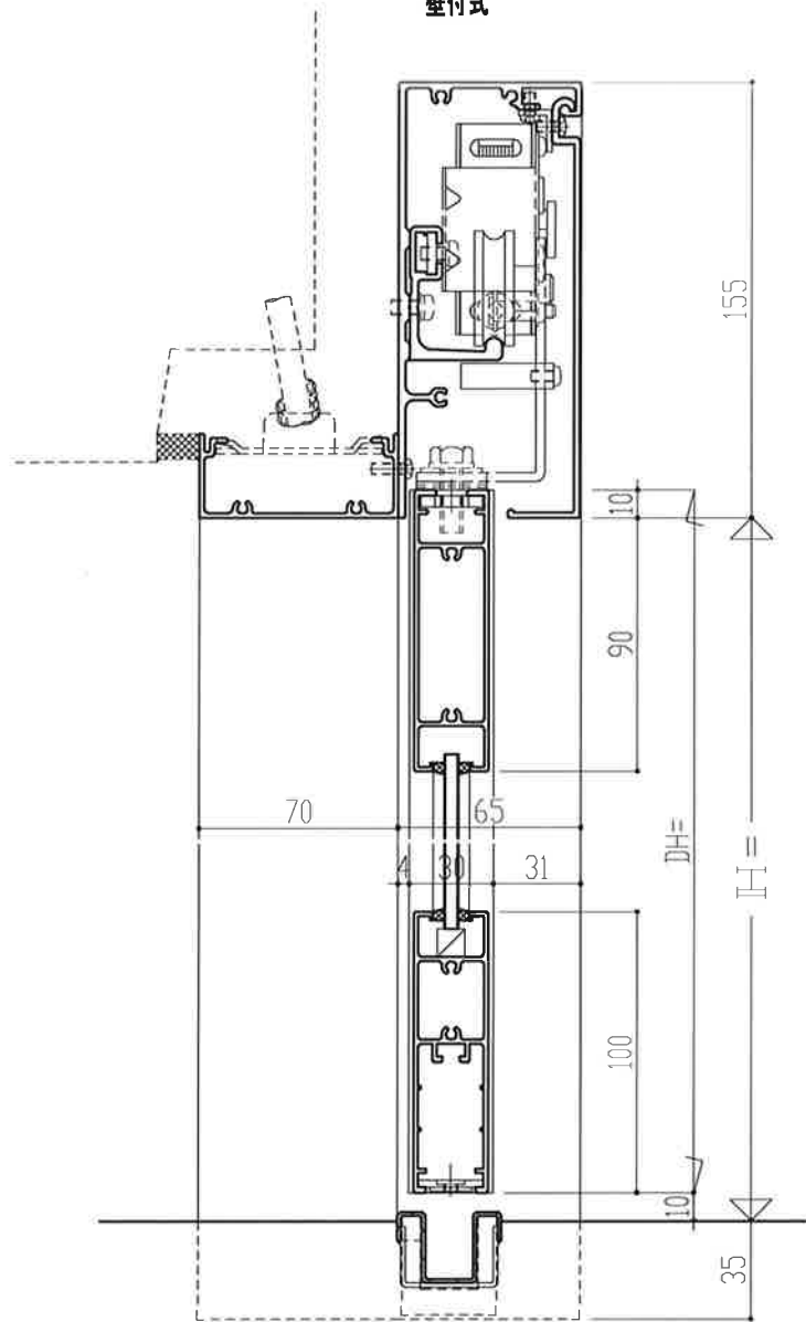
壁付式
