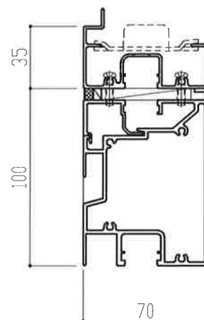
ALC納まり
