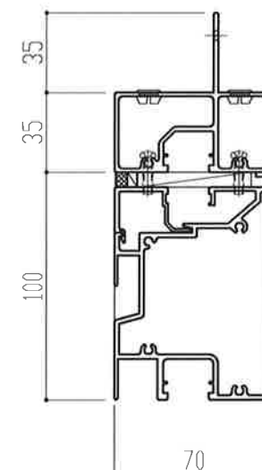
SC半外納まり
