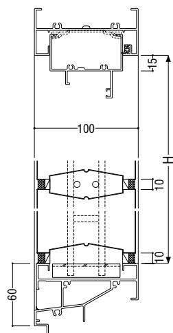
●外倒し排煙窓_RC枠
