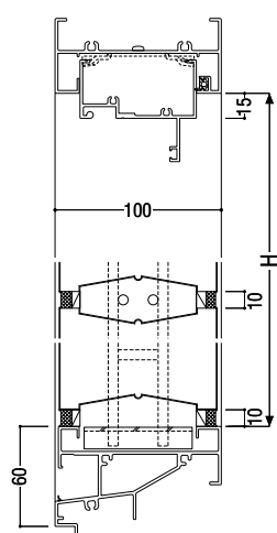
●突出し排煙窓_RC枠
