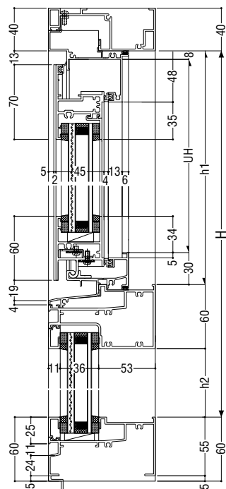
下枠納まり
