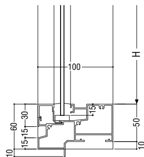
下枠納まり
