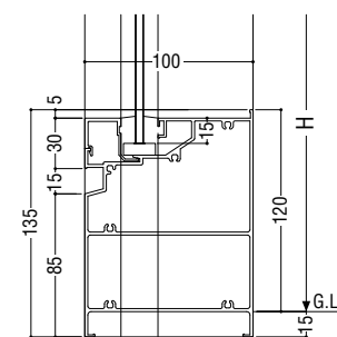
巾木納まり
