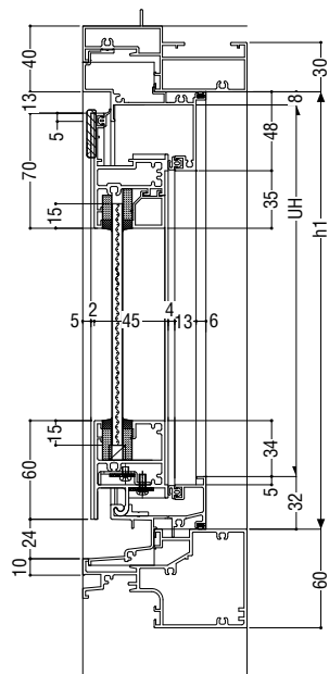
ランマ部
