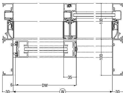
下段(開口部)納まり
