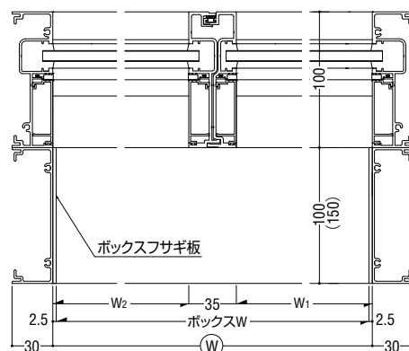
上段(FIX部)納まり
