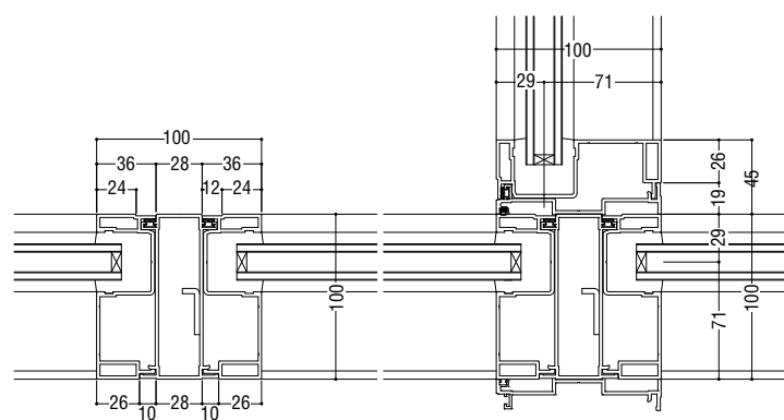
100mm見付汎用方立
