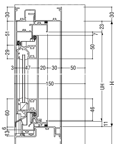
ハイH方立欄間部
