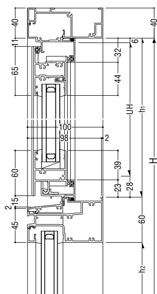
外倒し排煙窓-FIX窓
