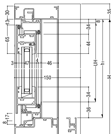
ハイH方立欄間部
