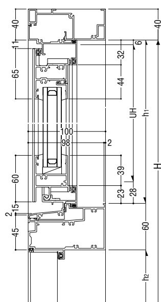
外倒し排煙窓-框ドア
