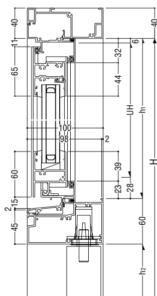
外倒し排煙窓-フロアヒンジドア
