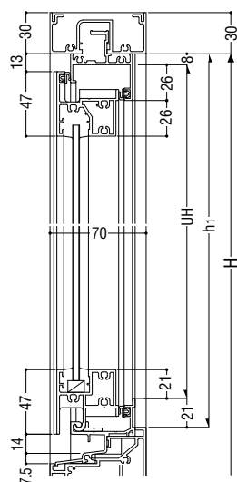
RC枠/Aタイプ
