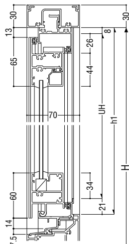
RC枠/Bタイプ
