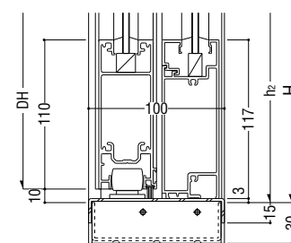
間仕切り型下枠
