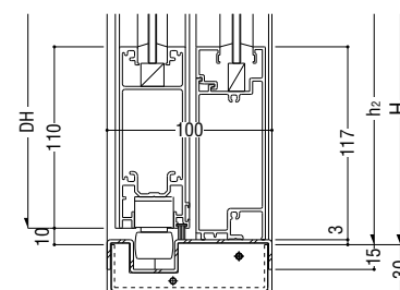
溝型下枠
