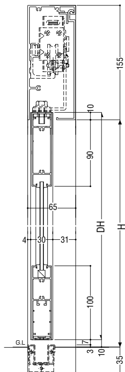
壁付式
