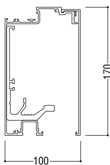
① 170mm見付無目
