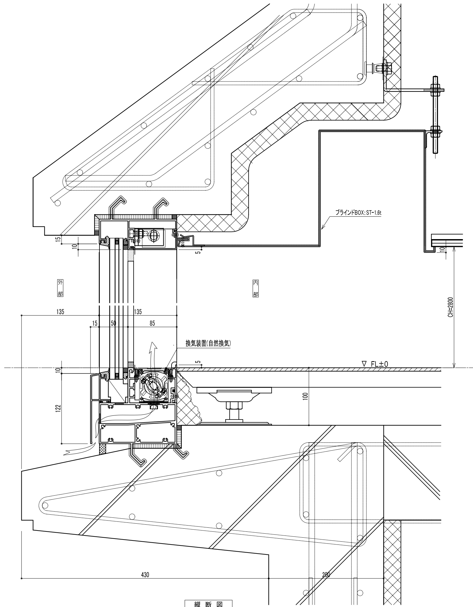
縦断図
