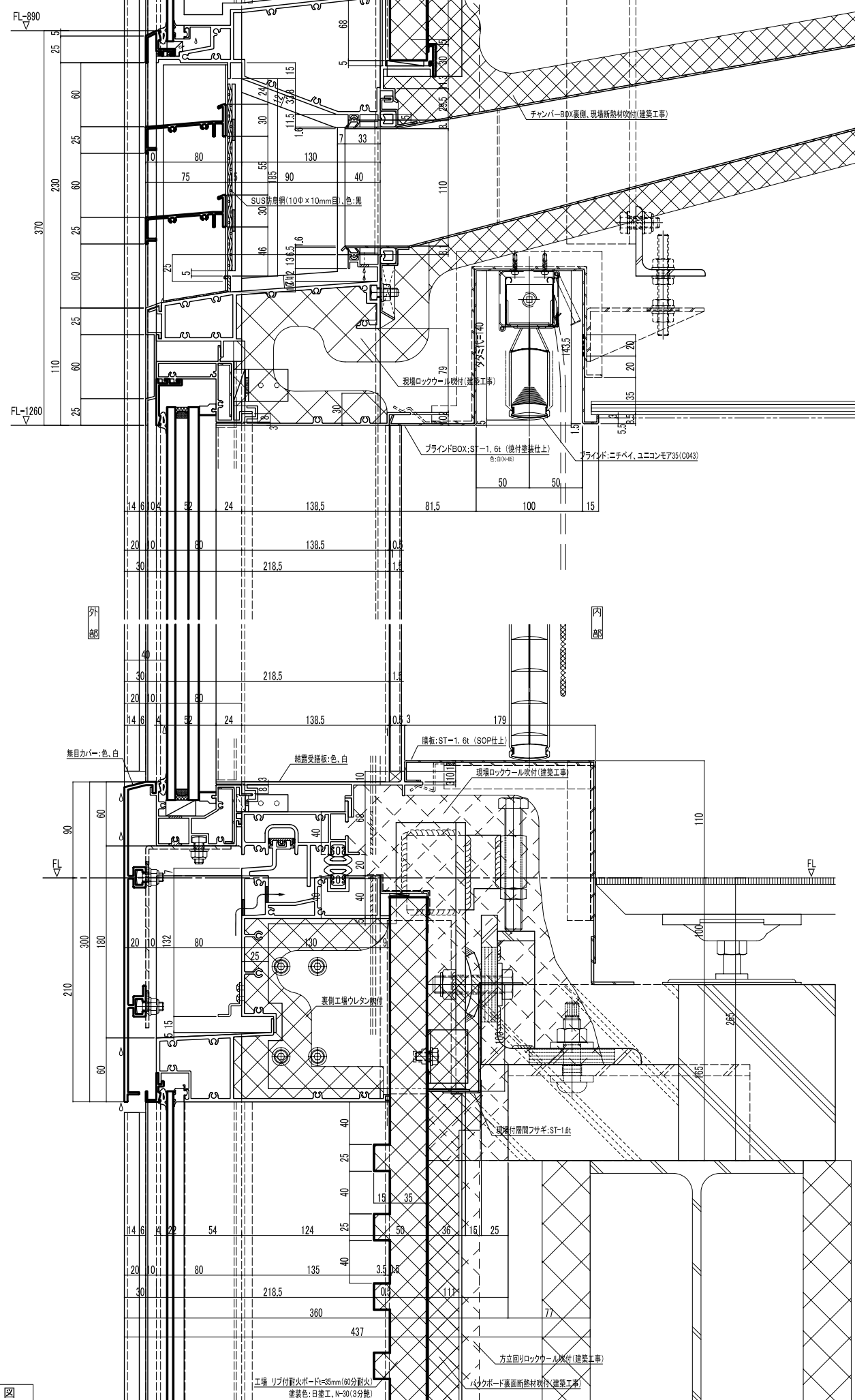
縦断図
