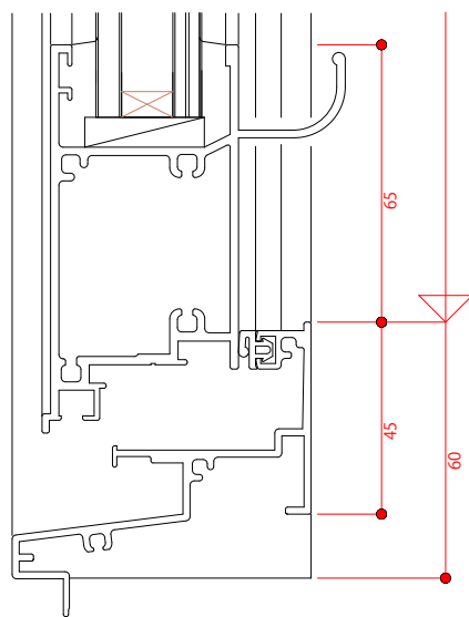
手架付下框
