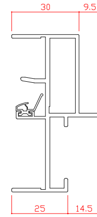
連窓方立が取付く 場合の縦枠
