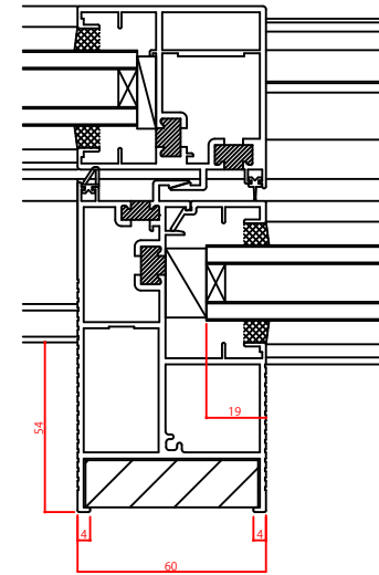
化粧木付き召し合せ框
