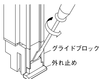
①はずれ止めの外し方
