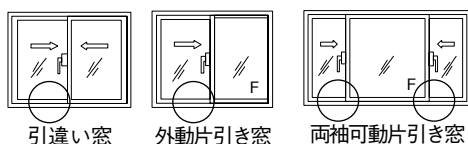
開口形式別取付位置
