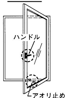
内開き窓
