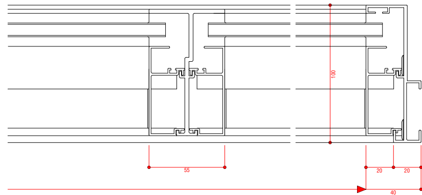
バックマリオンタイプ
