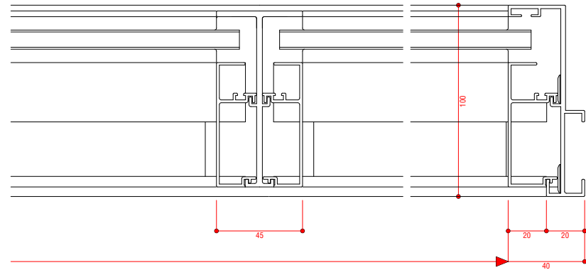
中間方立①
