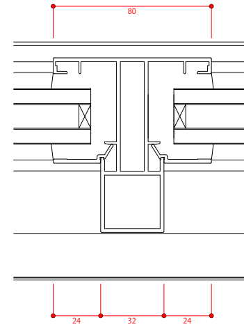
中間方立ZB
