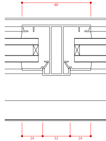
中間方立ZA
