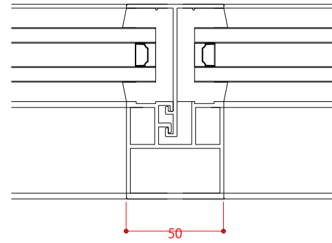
中間方立
