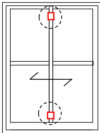
召し合せ枠部のみ
