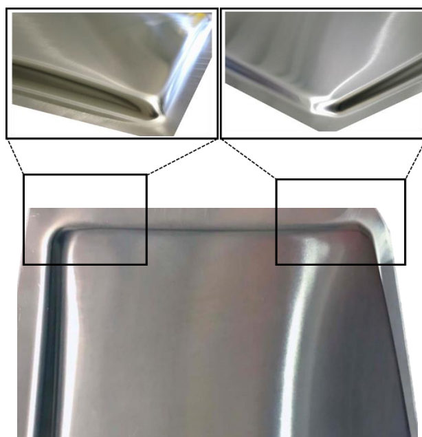
図4 室温プレスによる深絞り成形試作結果 小角形状（上部左図）、二段角形状（上部右図）
