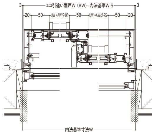
2枚建・4枚建共通 / 横断面
