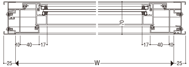
外動片引き窓(FNS-70)
