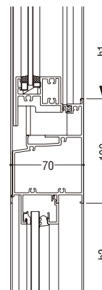
FIX窓(ガラス溝幅20mm)
