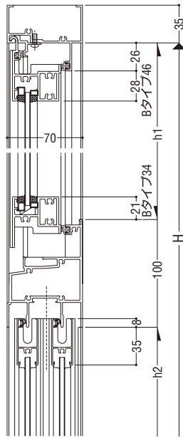
引違い窓(FNS-70)
