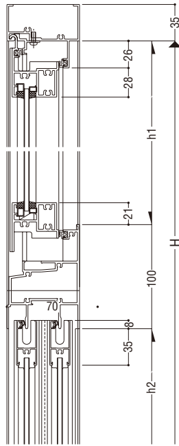
引違い窓(FNS-70)
