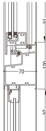
FIX窓(ガラス溝幅15mm)
