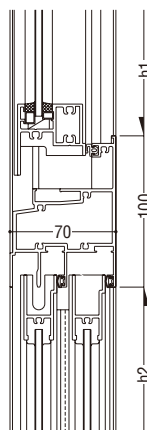
引違い窓(FNS-70AT)
