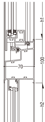
FIX窓(ガラス溝幅15mm)
