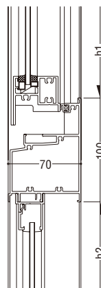
FIX窓(ガラス溝幅15mm)
