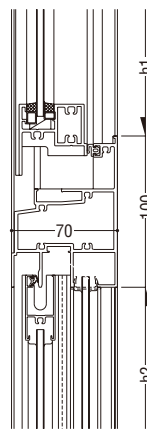
外動片引き窓(FNS-70)
