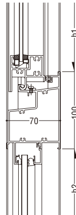
FIX窓(ガラス溝幅20mm)
