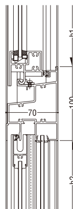
外動片引き窓(FNS-70)
