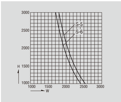
■無目耐風圧強度
