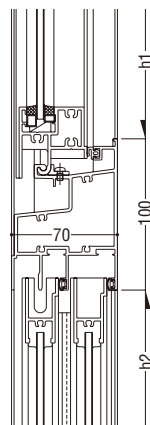
引違い窓(FNS-70AT)
