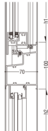
FIX窓(ガラス溝幅20mm)
