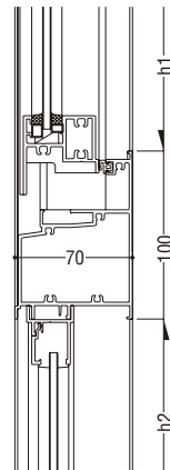
FIX窓(ガラス溝幅15mm) ※外押縁
