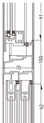
引違い窓(FNS-70AT)
