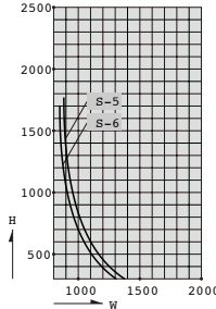
中棧③ (使用ガラス6mmを超える場合)
