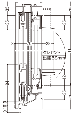
WDタイプ (FIX部20mm)
