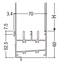
下枠外部アタッチを取付けない場合
