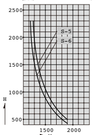
中棧Ⓑ (使用ガラス6mmを超える場合)
