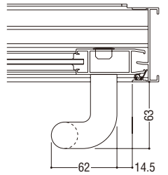
樹脂製把手 (標準装備外部品)
