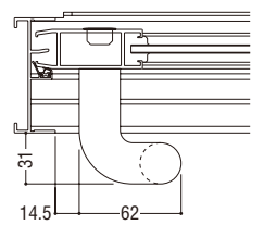
樹脂製把手 (標準装備外部品)
