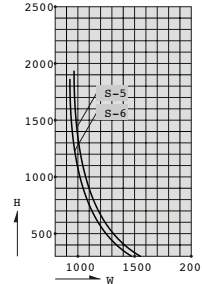
中棧④ (使用ガラス6mmを超える場合)
