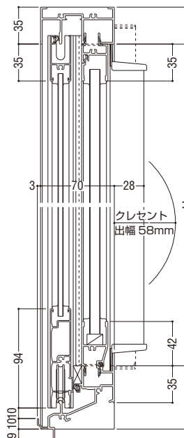
WDタイプ(FIX部20mm)
