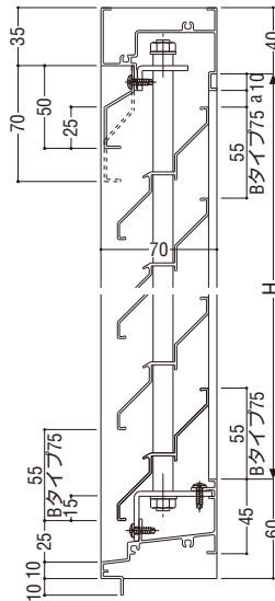
取りはずし式がらり
