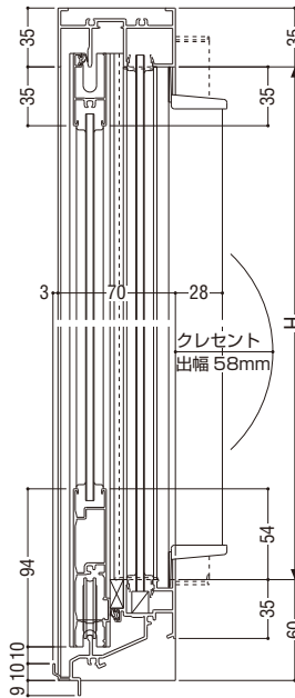
Dタイプ(FIX部15mm)
