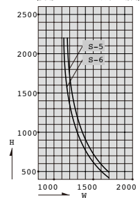
中棧② (使用ガラス6mm以下の場合)
