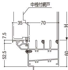
下枠外部アタッチ(35mm)を取付ける場合
