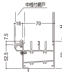
下枠外部アタッチ(18mm)を取付ける場合
