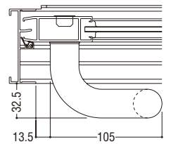
ステンレス製把手 (標準装備外部品)
