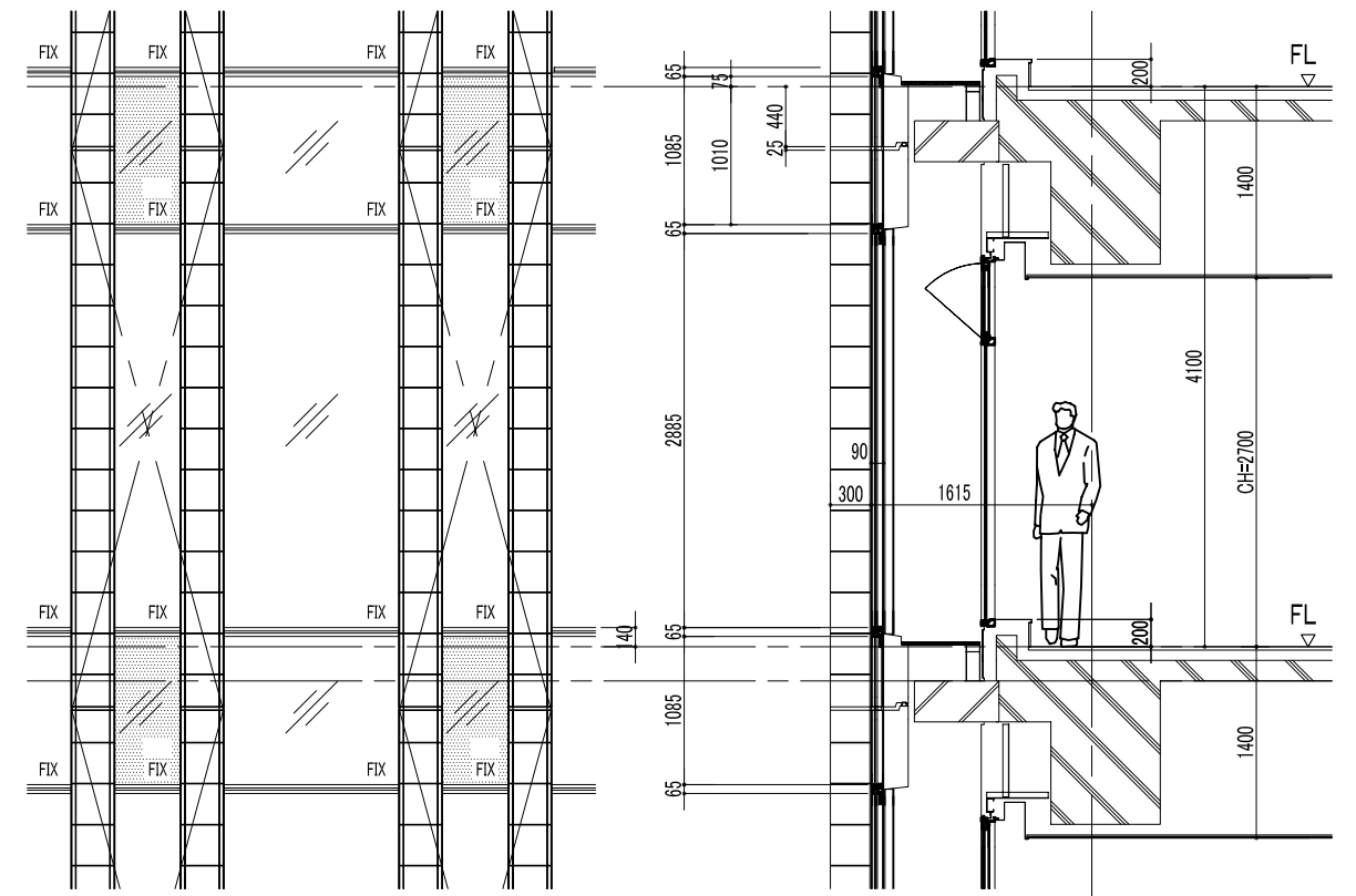
外観図
