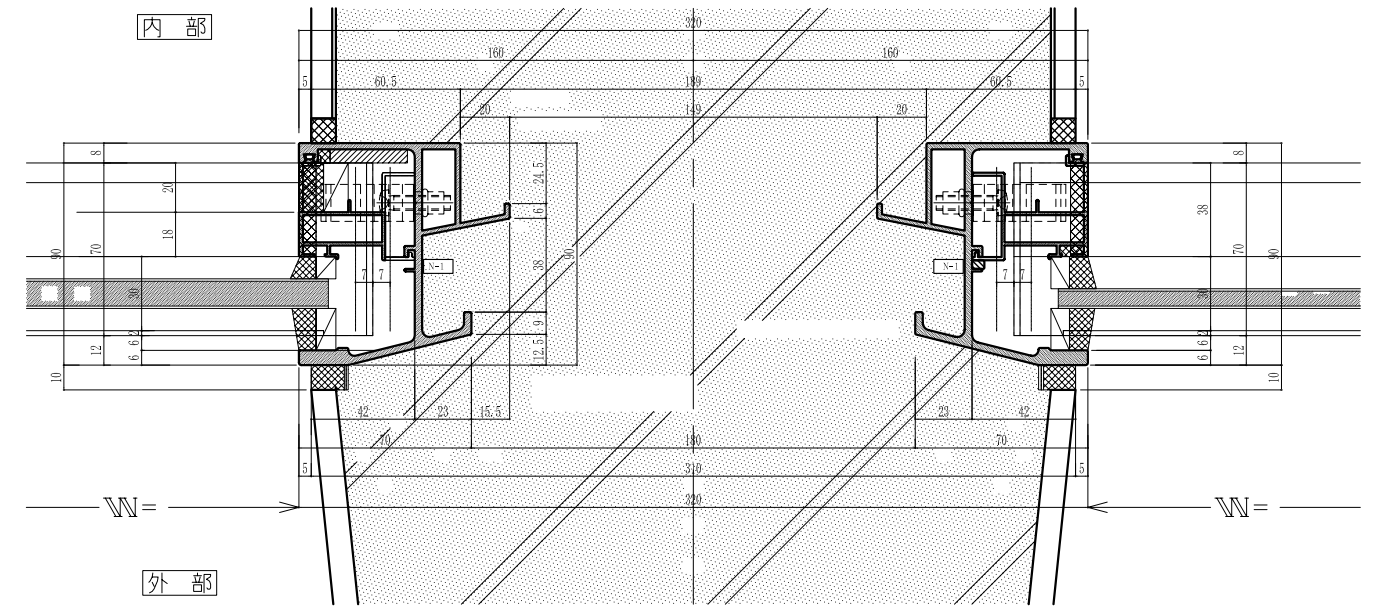
横断図
