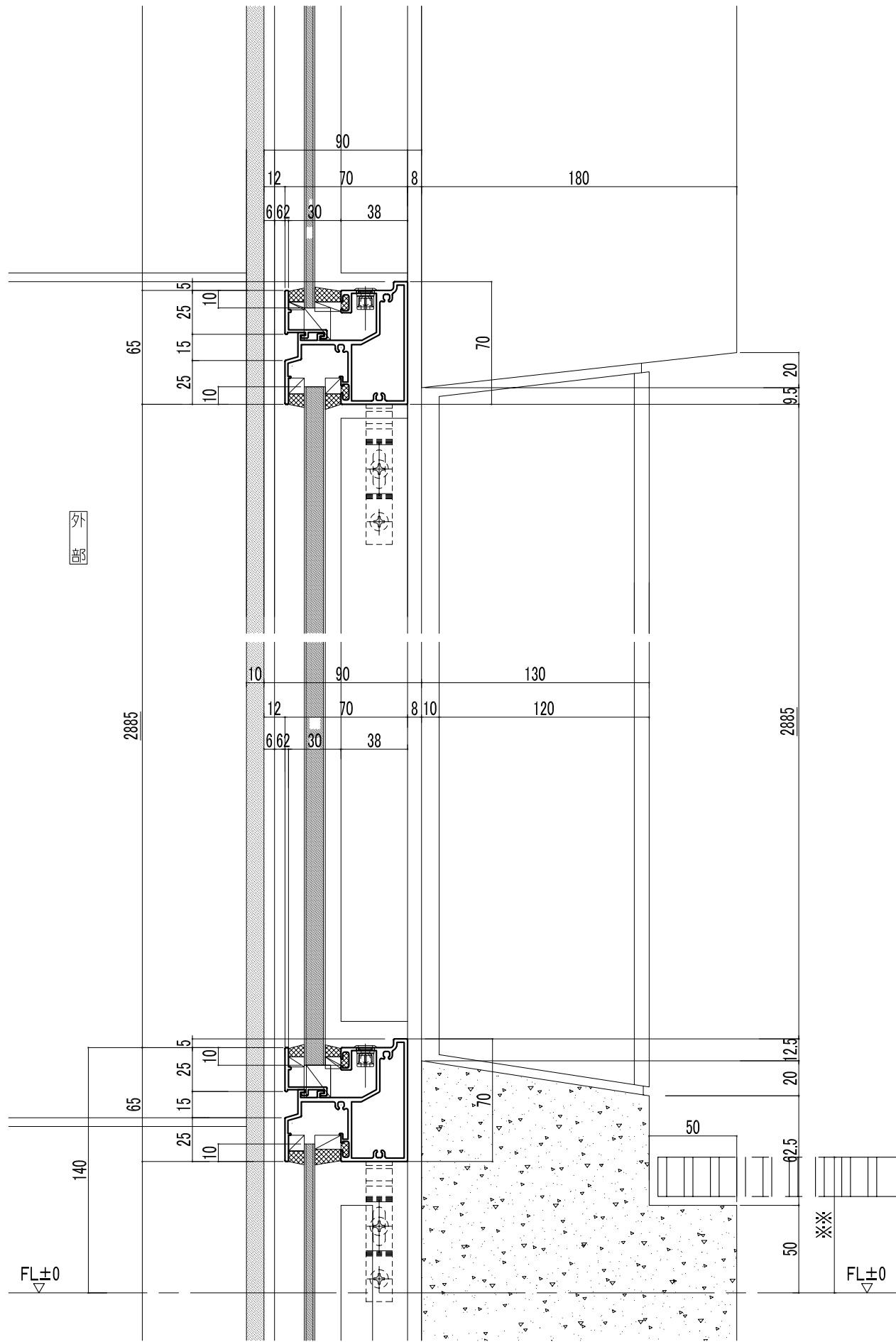
縦断図
