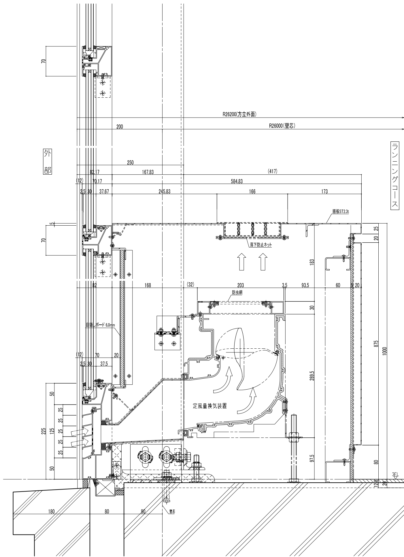
縦断図
